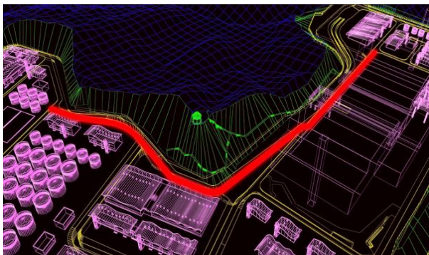
广州东部固体资源再生中心综合管廊
